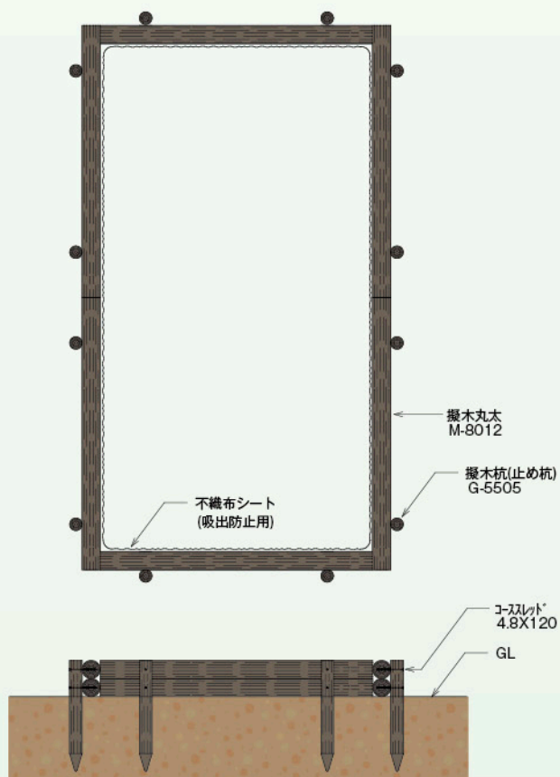
80φ擬木丸太と止め杭の組み合わせ参考図
