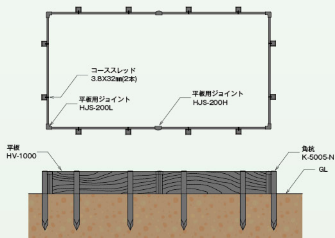
角杭と平板の組み合わせ参考図
